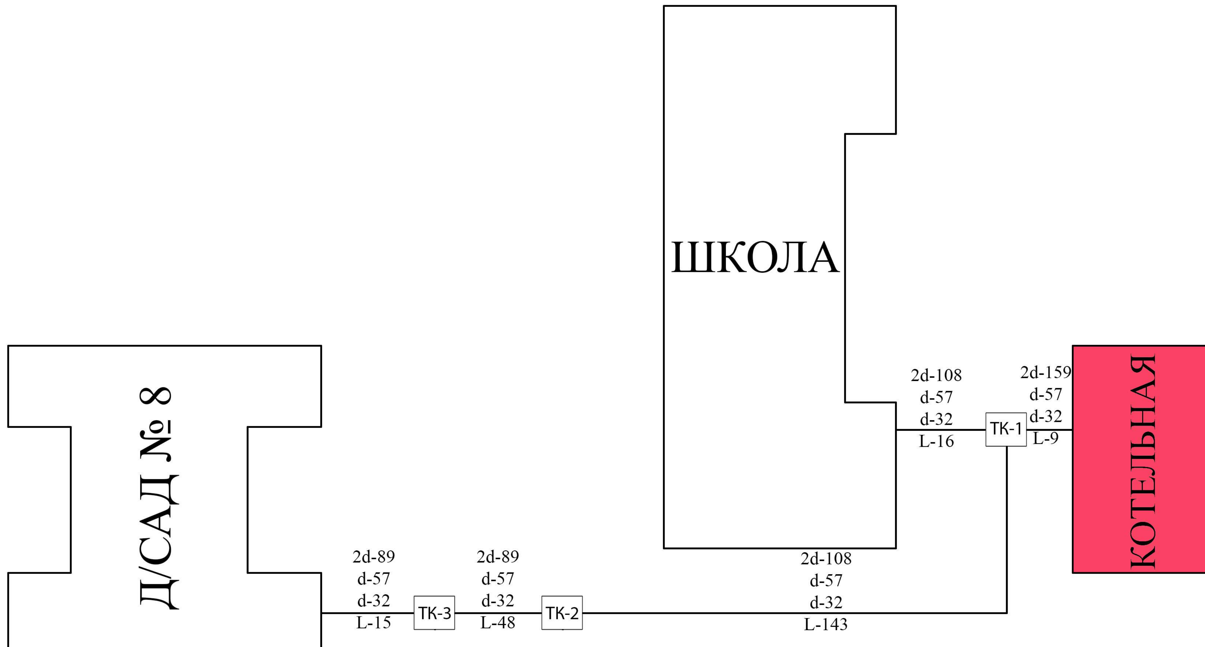
Схема теплоснабжения городского округа Баксан
